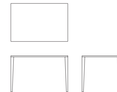
6003 - 6103 L.120cm P.80cm H.76cm W.47 1/4" D.31 1/2" H.30"
