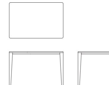
5002 - 5102 L.120cm P.80cm H.76cm W.47 1/4" D.31 1/2" H.30"
