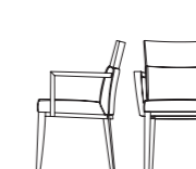
00933 L.61,5cm P.58cm H.86,5cm H.s.48cm H.b.66cm W.24 1/4" D.22 3/4" H.34" S.h.19" A.h.26"
